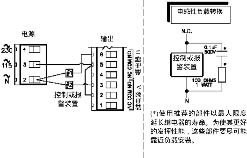
图 2-6 连接控制/报警装置与继电器
